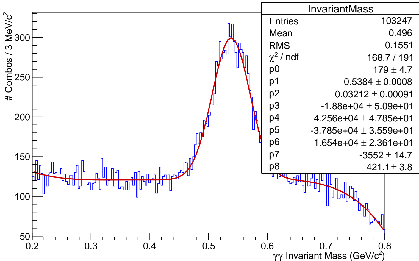
Reconstructed Eta - Spring 2015 Data (2931, 3079, 3179, 3180, 3185, 3186)
