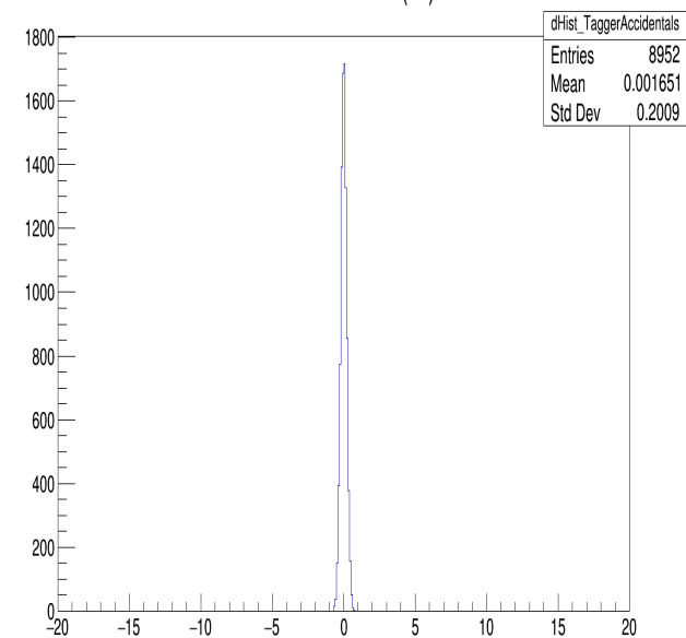
Vertex time - RF (ns)
