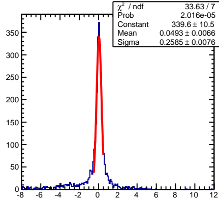
E = 1.0-1.5 GeV
