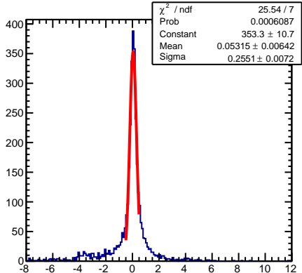
E = 0.8-1.0 GeV
