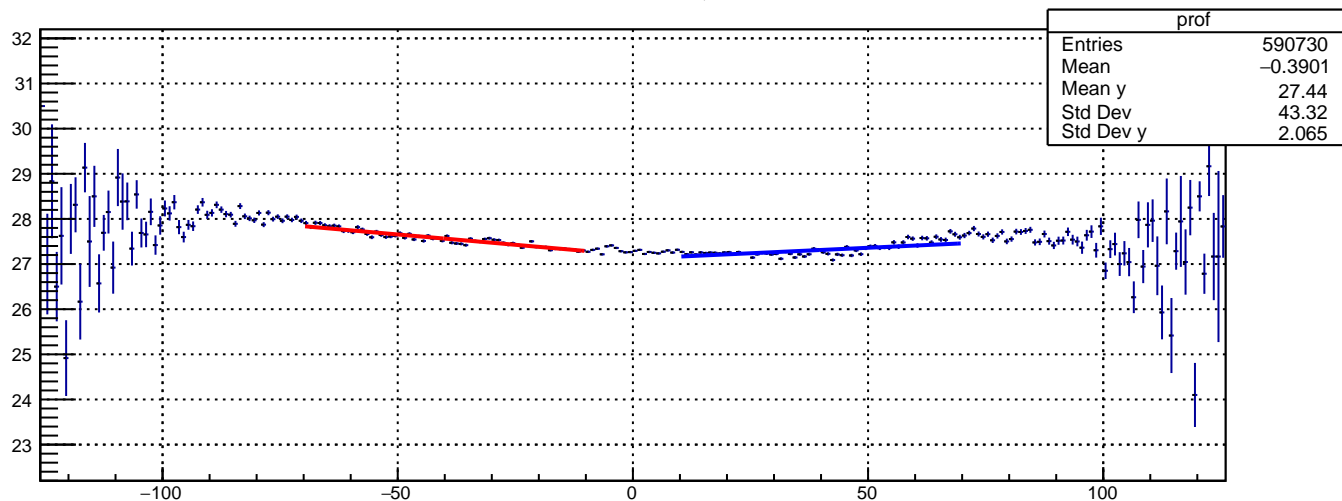
HorizontalPlaneQP27
