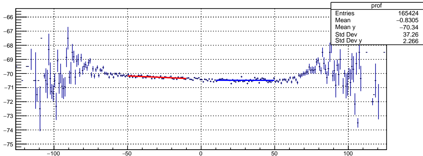
HorizontalPlaneQM9
